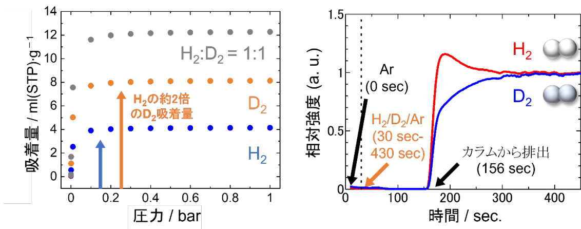
図 2. IAST 理論から予測される選択的な D 2 の吸着挙動(左)、および 破過実験(40°C)における特異的な H 2 /D 2 分離能(右)
